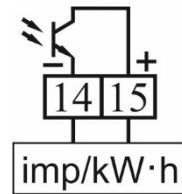
Рисунок Б. 2. Схема підключення основного випробувального виводу
