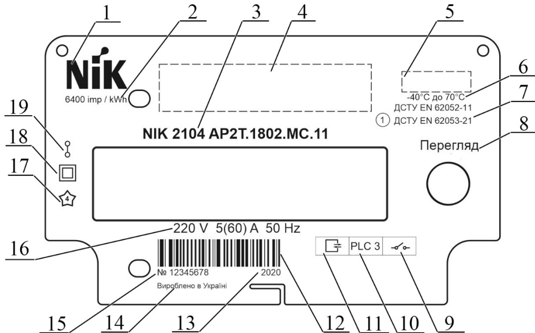
Рисунок 5. Дизайн паспортної таблички для РКІ варіанту 2
