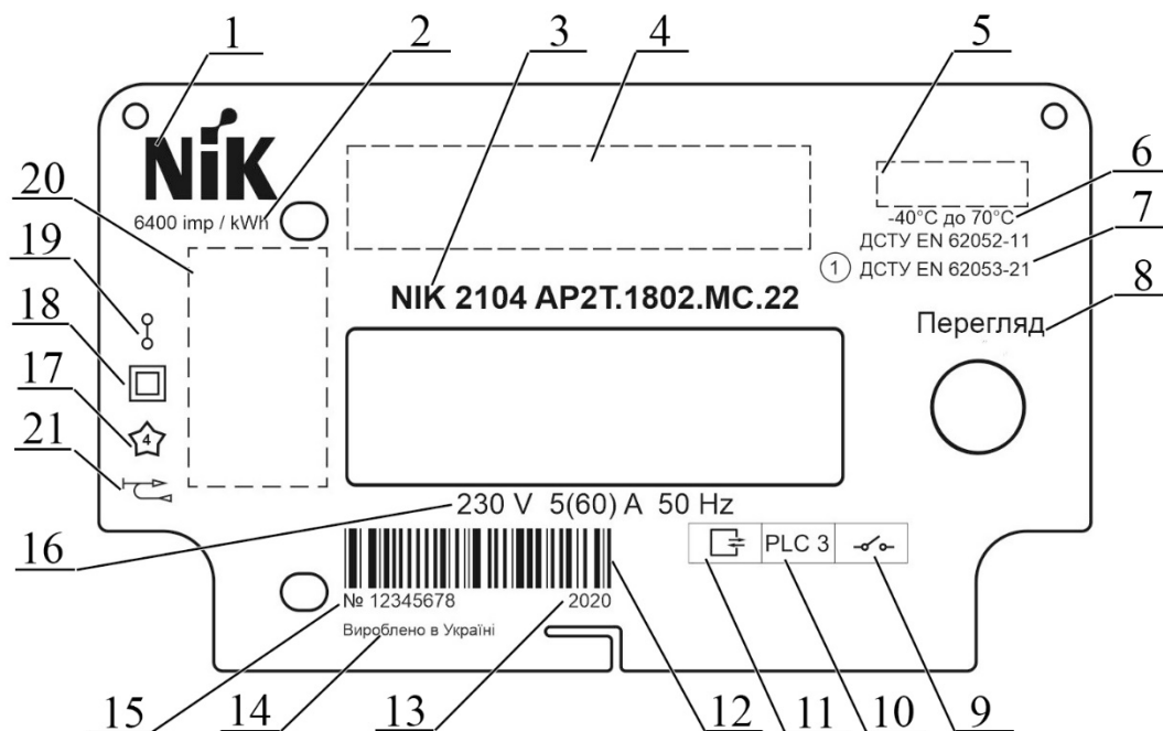
Рисунок 4. Дизайн паспортної таблички для РКІ варіанту 1
