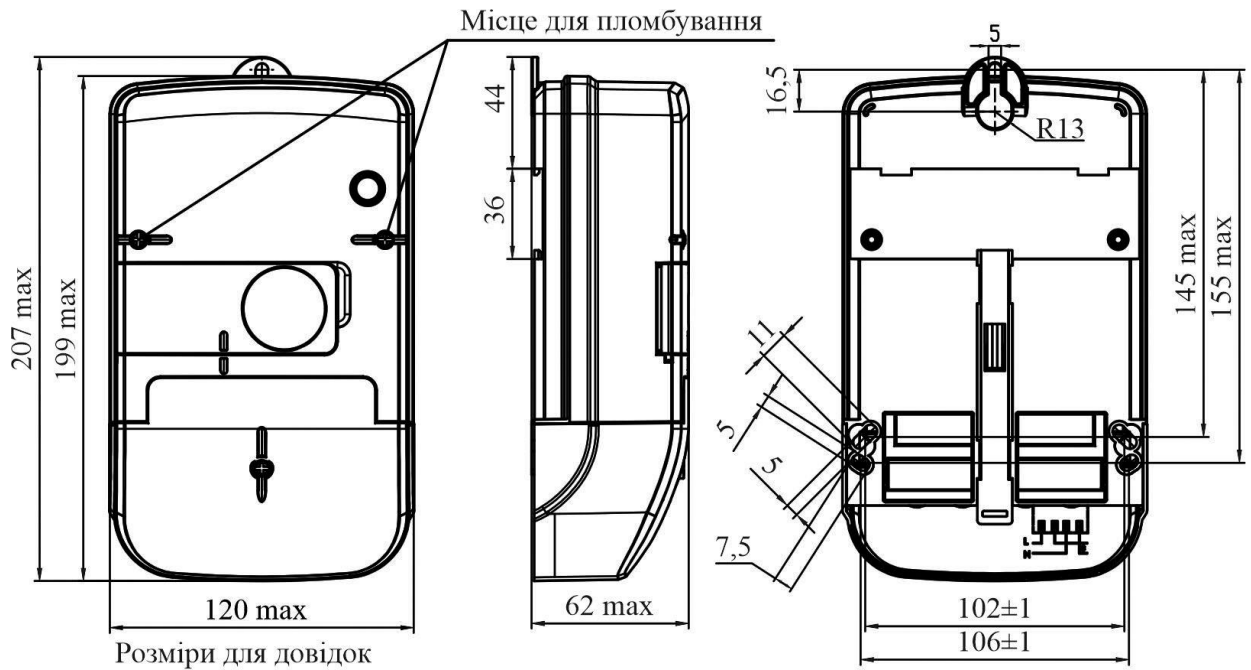
Рисунок А. 1. Габаритні та встановлювальні розміри лічильників
