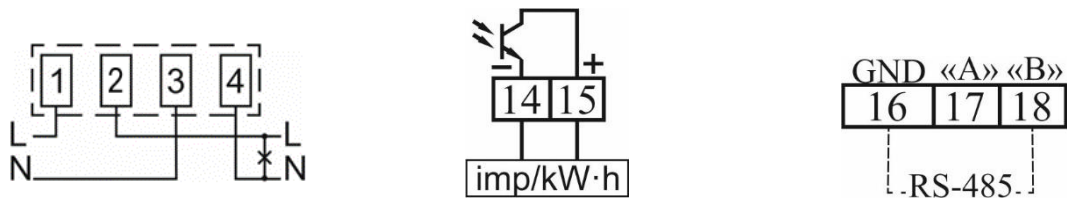
Рисунок 1. Схема підключення лічильника
