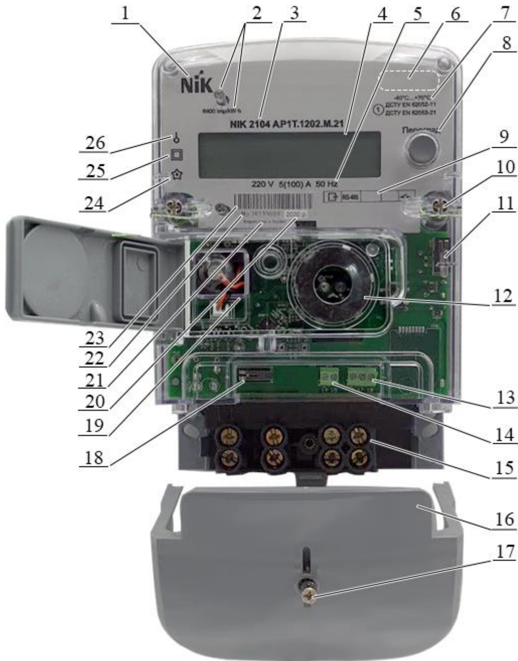
Рисунок 1. Зовнішній вигляд лічильника типу 2104 ...P1...
